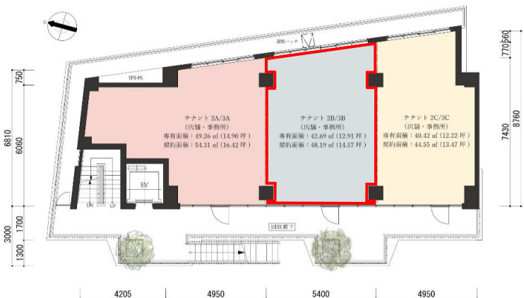
【2/3階平面図】
