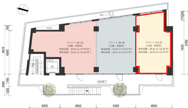
【2階平面図】
